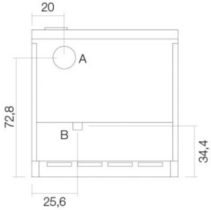
posteriore - back - postérieur - hinter
